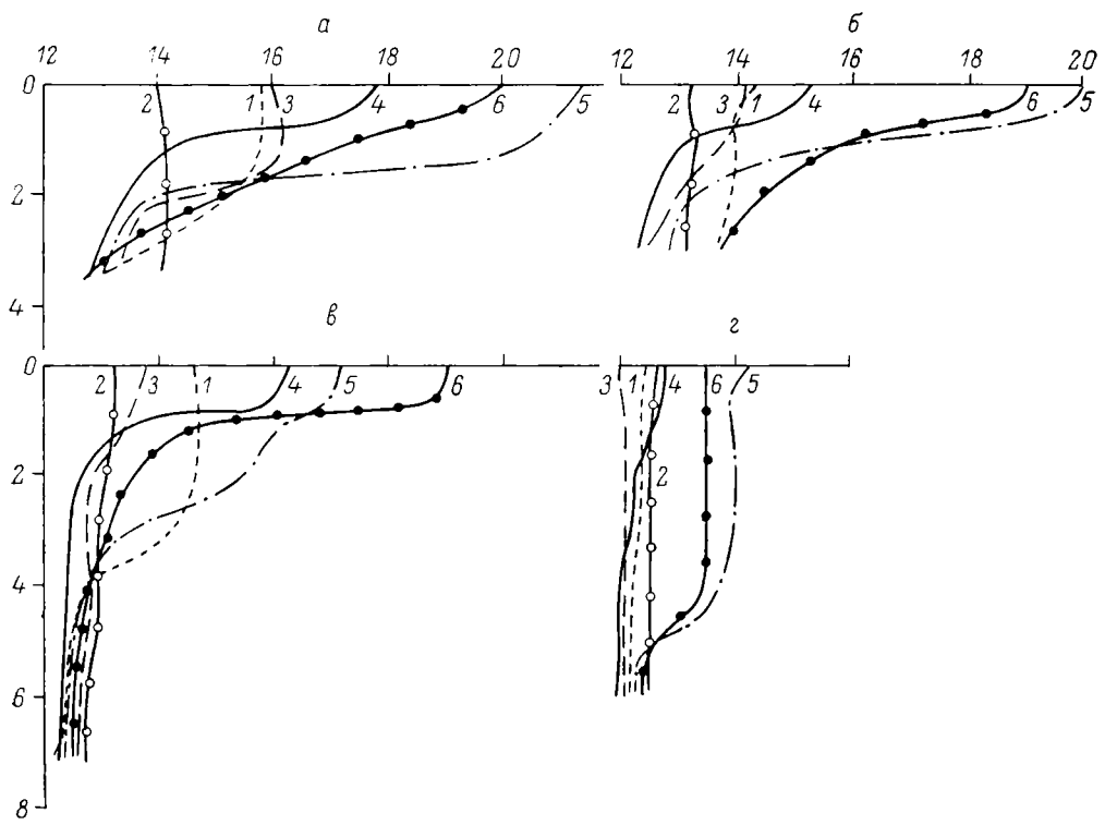
Рис. 27. Характерные кривые распределения температуры воды по глубине в Ивановском водохранилище в зоне влияния подогретых вод Конаковской ГРЭС (а—б) и вне этой зоны (в, г). 1—6 — номера серий наблюдений. По оси ординат — глубина, м, по оси абсцисс — температура, °С.
