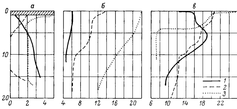
Рис. 26. Характерные кривые распределения температуры воды по глубине. а — в период ледостава (Рыбинское водохранилище): 1 — 23 марта 1962 г., 2 — 20 апреля 1960 г., 3 — 20 апреля 1950 г. б — в безледный период при обычных условиях накопления тепла (Рыбинское водохранилище): 1 — 28 мая 1956 г., 2 — 26 мая 1954 г., 3 — 19 июня 1954 г. в — в безледный период при различных погодных условиях: 1 — 31 мая 1954 г. (Рыбинское водохранилище), 2 — 16 июня 1959 г. (Горьковское водохранилище), 3 — 10 июня 1956 г. (Рыбинское водохранилище). По оси ординат — глубина, м, по оси абсцисс — температура, °С.
